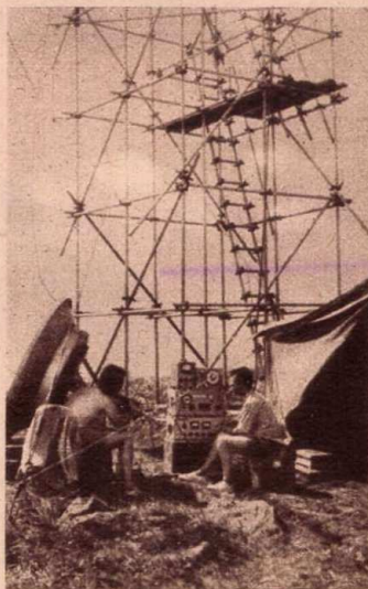
Mikrohullámú mérések szabad terepen
